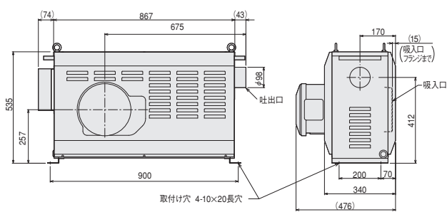
HAP2103T
