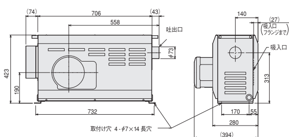
HAP2053T
