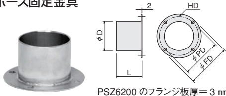
PSZ6200 のフランジ板厚 = 3 mm
